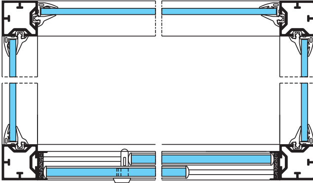
MOBILIER VITRINE AVEC PORTE COULISSANTE
