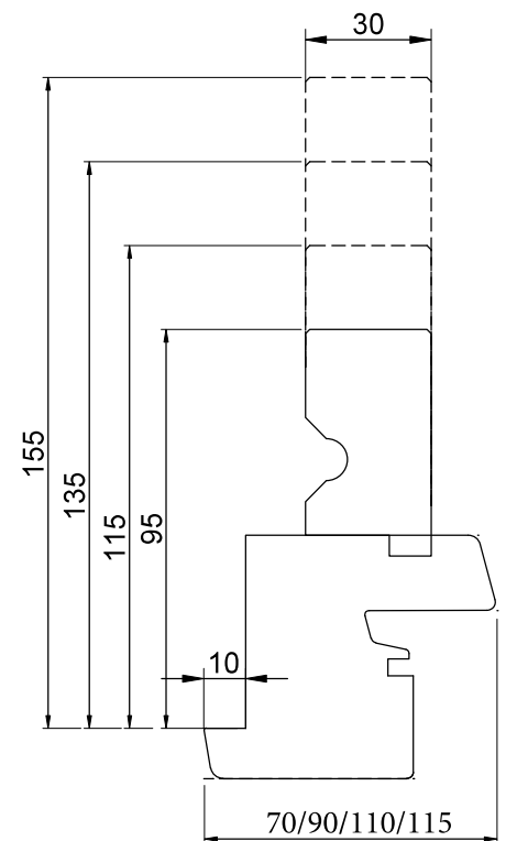
Dormant Neuf avec aile 70*58 avec fausses tapées pour doublage
