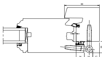
Fiche broche 12/82
