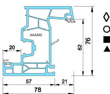
Ouvrant dans l'ouvrant 78mm
