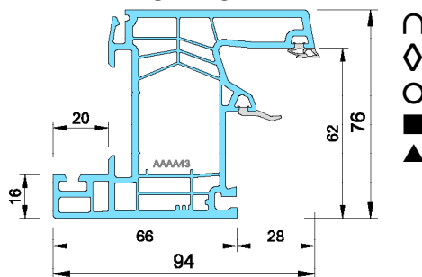
Dormant Neuf avec aile 94*76
