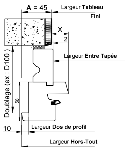
Cas N°1 (par défaut sans VR)
