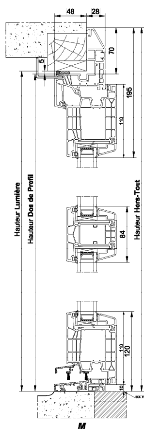
Rénovation Aile de 70mm
