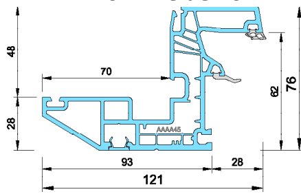
Dormant Rénovation 121*76 - Aile de 70mm
