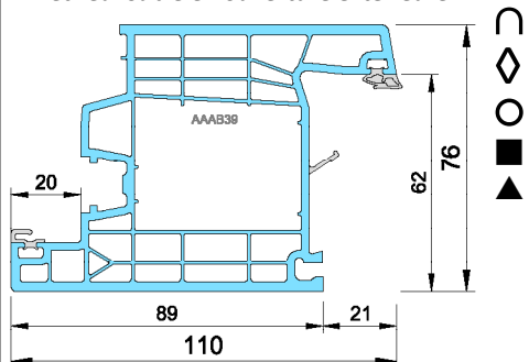
Ouvrant de 110mm Ouverture intérieure et réalisable en ouverture extérieure
