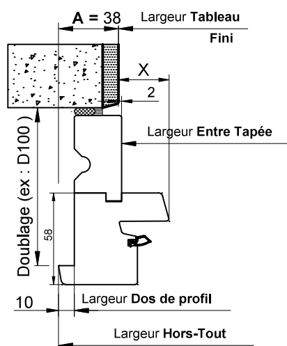
Cas N°2 (Obligatoire avec VR)
