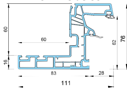
Dormant Rénovation 111*76 - Aile de 60mm
