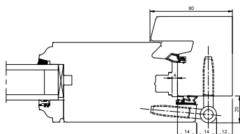
Fiche réglable 3D
