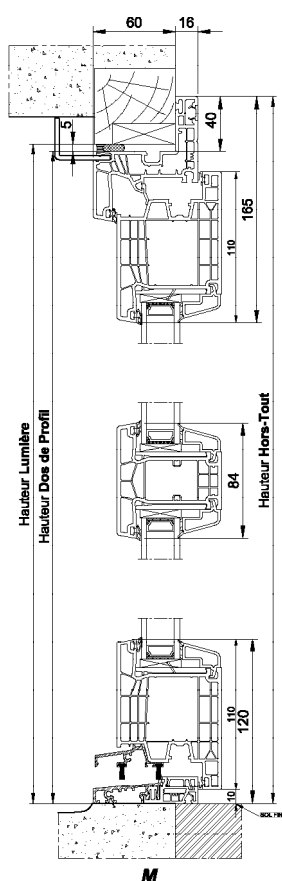
Rénovation Aile de 40mm
