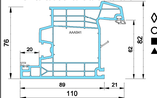
Ouvrant de 110mm Ouverture intérieure non réalisable en ouverture extérieure
