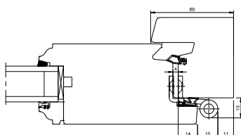
Paumelle entaillée
