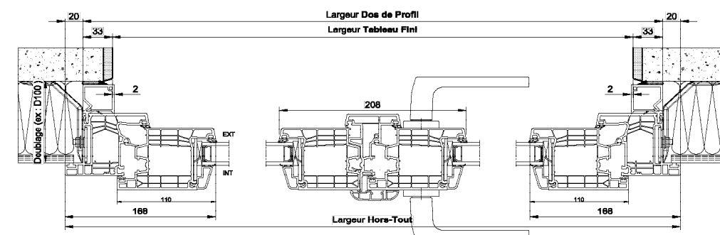
Neuf avec aile + tapées Aile de 20mm
