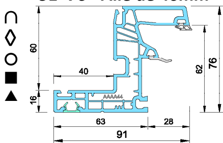
Dormant Rénovation 91*76 - Aile de 40mm
