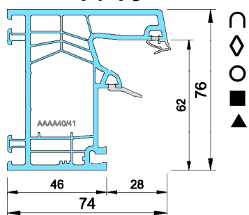
Dormant Neuf sans aile 74*76
