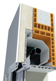
DEMI-LINTEAU OPTIBLOC
