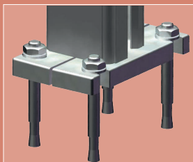
Platine à visser pour claustra de 1800 mm
